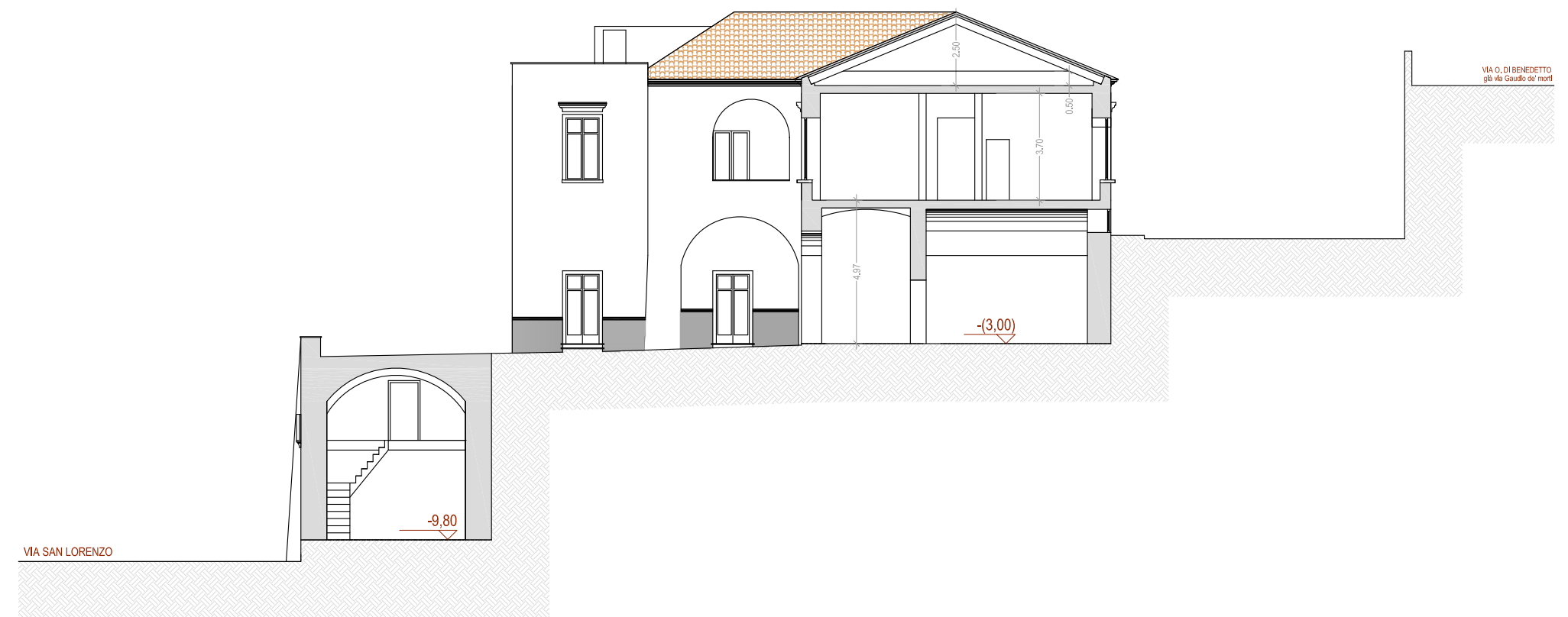
SEZIONE D-D'
